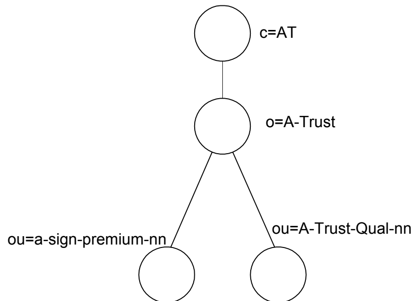
Abbildung 2 Verzeichnisbaum
